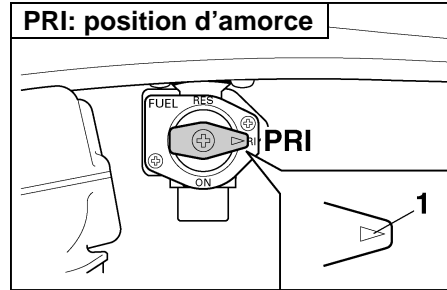
1. Flèche placée sur "PRI"
